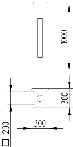
Fundament FS100
